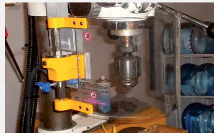
PROTEZIONI PER TRAPANI GUARDS FOR DRILLING MACHINES
