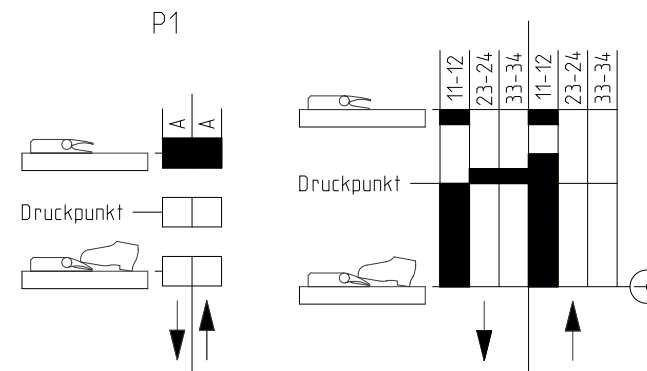
Beispiel eines Schalt diagrammes für einen Zustimmungsschalter mit zusätzlicher Positionserkennung (Ausgang A)
